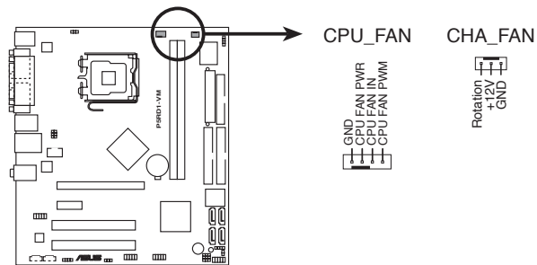
P5RD1-VM Fan connectors
